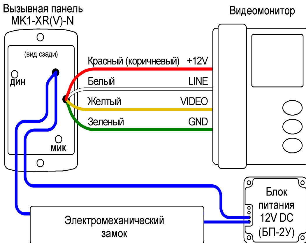
Рис 1. Подключение блока вызова МК1-ХRV-N
